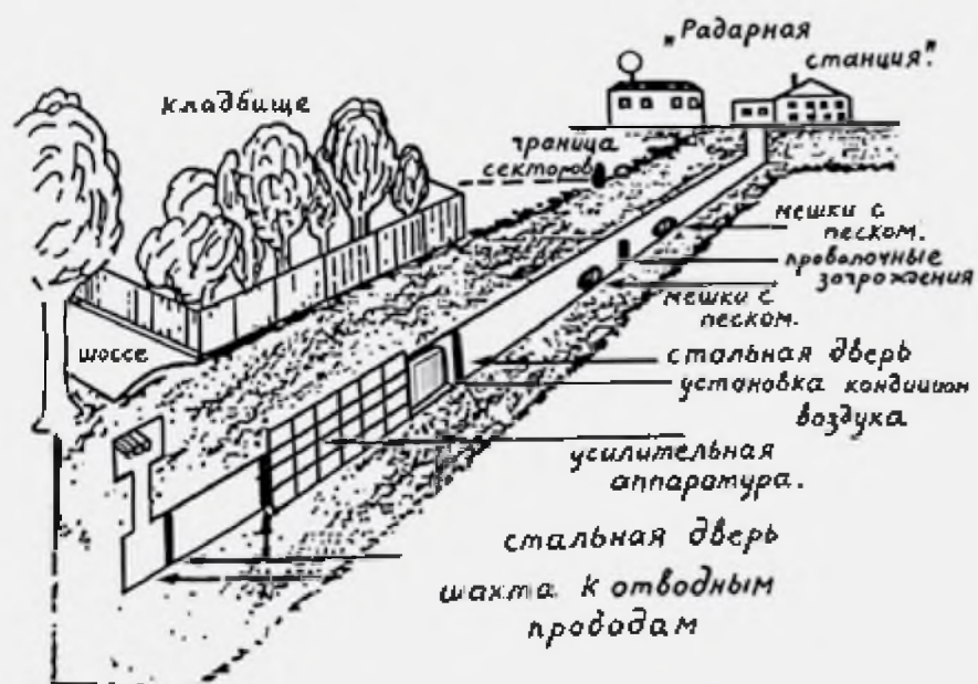
План-схема Берлинского туннеля из архива СВР России
